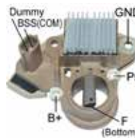
VRH2009-164 Mitsubishi, Renault
