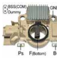
VRH2009-160 Mitsubishi, Citroen, Peugeot, Skoda
