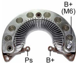
Heat Sink(+) Bottom
